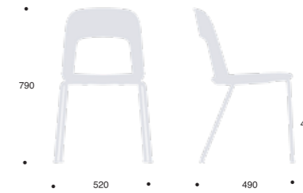
四脚椅 (HFF060)
